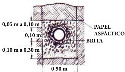
CORTE TRANSVERSAL DA VALA
