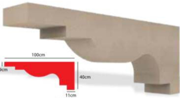
PY-07 Payanda / Klasik
