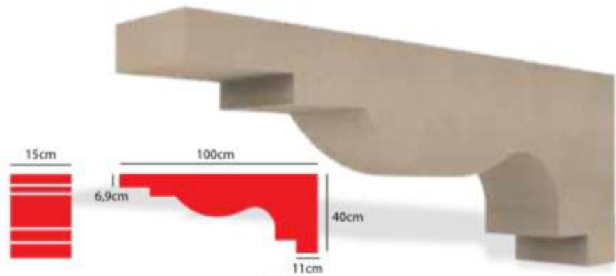
PY-07 Payanda / Klasik
