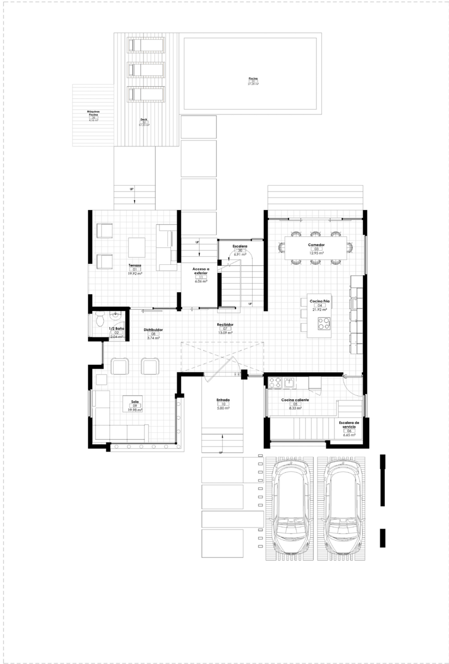
1 PLANTA ARQ. AMUEBLADA 1ER NIVEL
