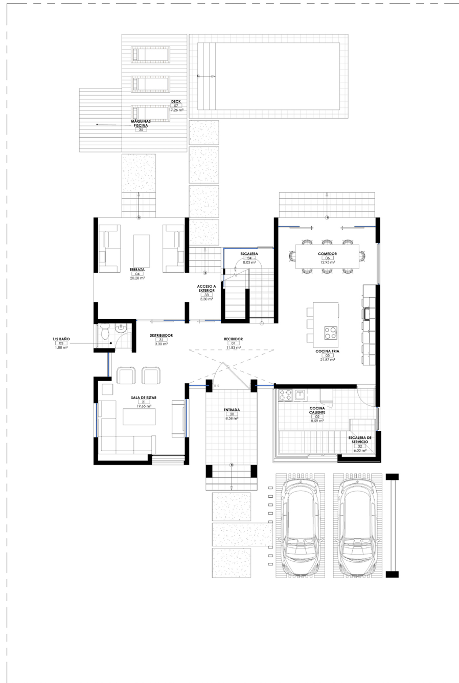
1 PLANTA ARQ. AMUEBLADA 1ER NIVEL 1:60
